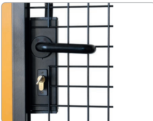
Cod. PS-SERR Chiusura standard con chiave per scorrevole
